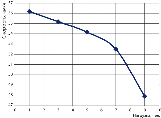
Результаты замеров скорости моторолки «Диана-4» под ПМ Mercury 60
